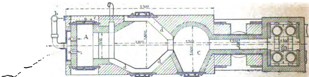
Fig. 93-94. — Four de puddlage au gaz de tourbe.
